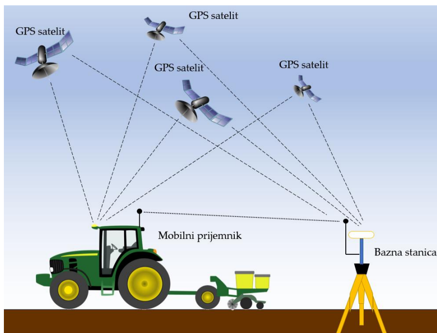
Slika 2.13. Komunikacija u slučaju RTK korekcije položaja korišćenjem bazne stanice
