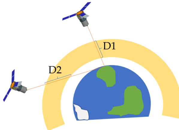
Slika 2.4. Prikaz različitog uticaja atmosfere na degradaciju signala za različite pozicije satelita u odnosu na prijemnik
