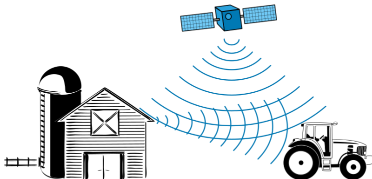
Slika 2.5. Ilustracija odbijanja GPS signala od objekta koji se nalaze u blizini prijemnika
